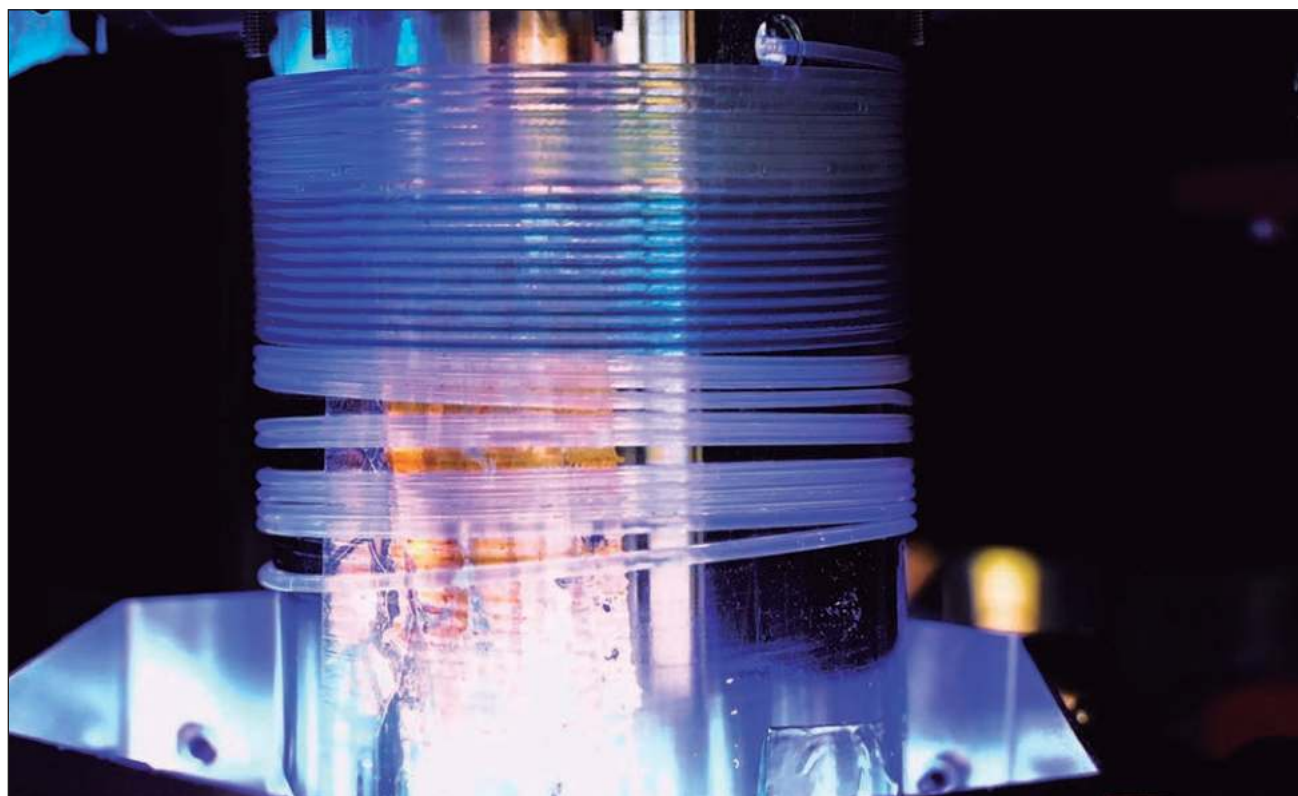
▲ El estudio muestra que el robot es un químico preciso y confiable que puede realizar una variedad de reacciones mientras produce cantidades mínimas de desechos, ofreciendo resultados de forma rápida e incansable. Foto UVA/HIMS
