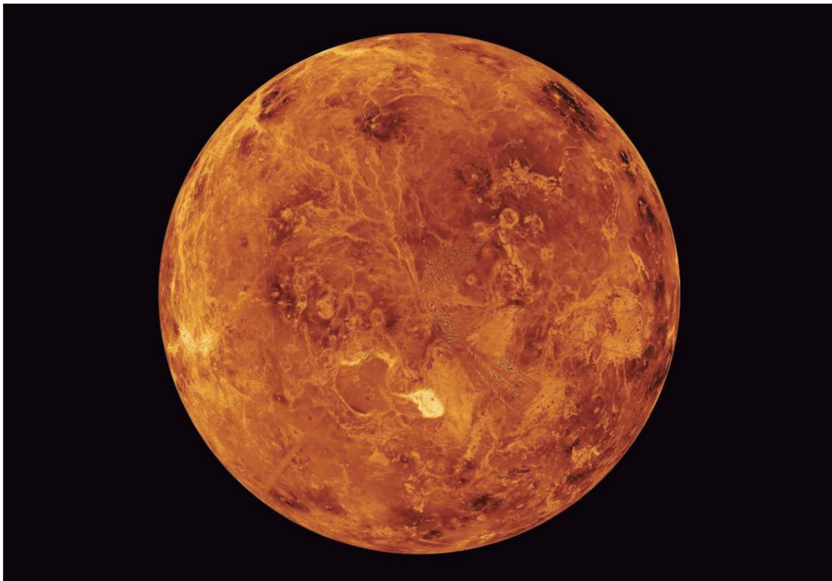
▲ Se trata de una enorme estructura creada por un impacto que contiene múltiples anillos, el más externo tiene un diámetro de mil 500 kilómetros. Foto NASA
