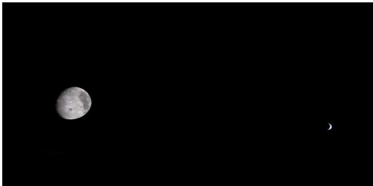
▲ Al salir de detrás de la Luna, vivieron un eclipse solar total, ya que el astro bloqueó el Sol desde su perspectiva. Foto NASA
