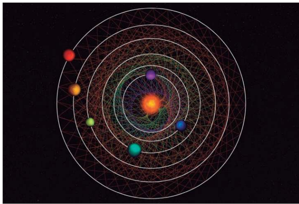
▲ Este sistema solar es único porque los seis planetas se mueven de manera similar a una sinfonía; en términos técnicos, se conoce como resonancia que es precisa, explicó el coautor Enric Palle, del Instituto de Astrofísica de Canarias. Foto ESA Thibaut Roger/NCCR PlanetS
