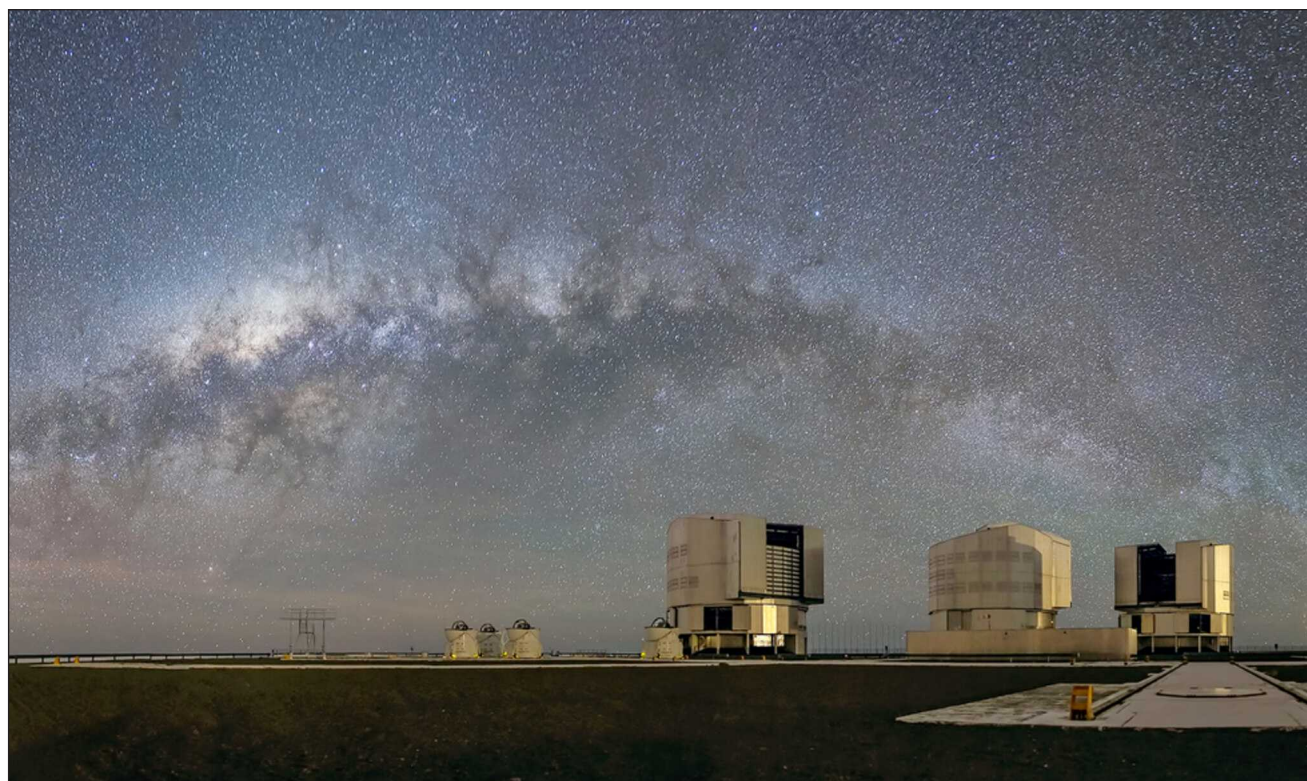
▲ El cuerpo celeste recién descubierto también orbita el agujero negro a una distancia más cercana de lo que los científicos habían visto nunca, y tarda apenas 8.7 años en completar una revolución. Foto ESO / John Colosimo
