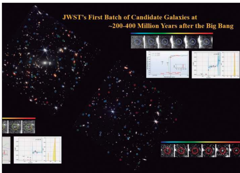
▲ El descubrimiento de Edwin Hubble de que el universo está en constante expansión es clave para comprender cómo se usan los desplazamientos al rojo en astronomía. Foto NASA/ESA/CSA
