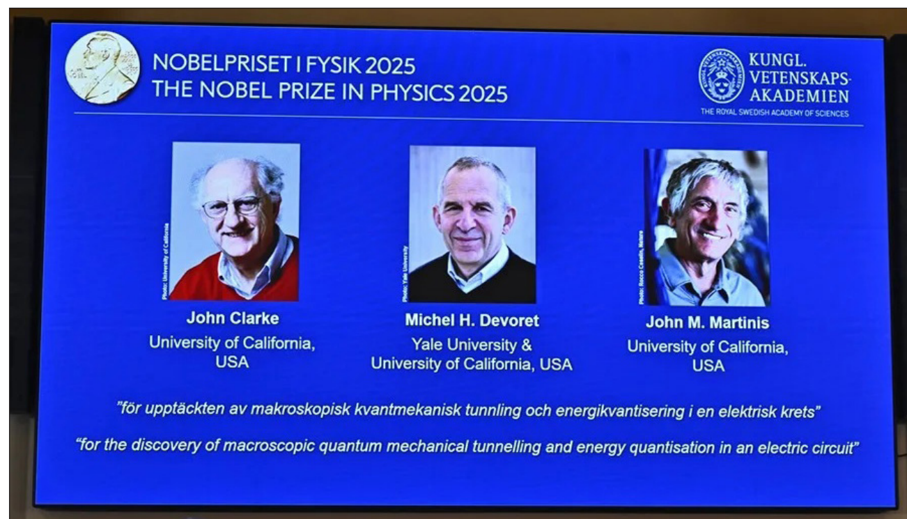
▲ El fallo de la Real Academia Sueca de Ciencias resalta "el descubrimiento del efecto túnel cuántico macroscópico y la cuantización de la energía en un circuito eléctrico", que se aplican ya en muchos teléfonos móviles, por ejemplo. Foto Efe
