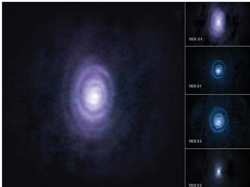
▲ Los expertos no descartan que la presencia de una estrella cercana influya en la manera en que V Hya se extingue. Foto ALMA
