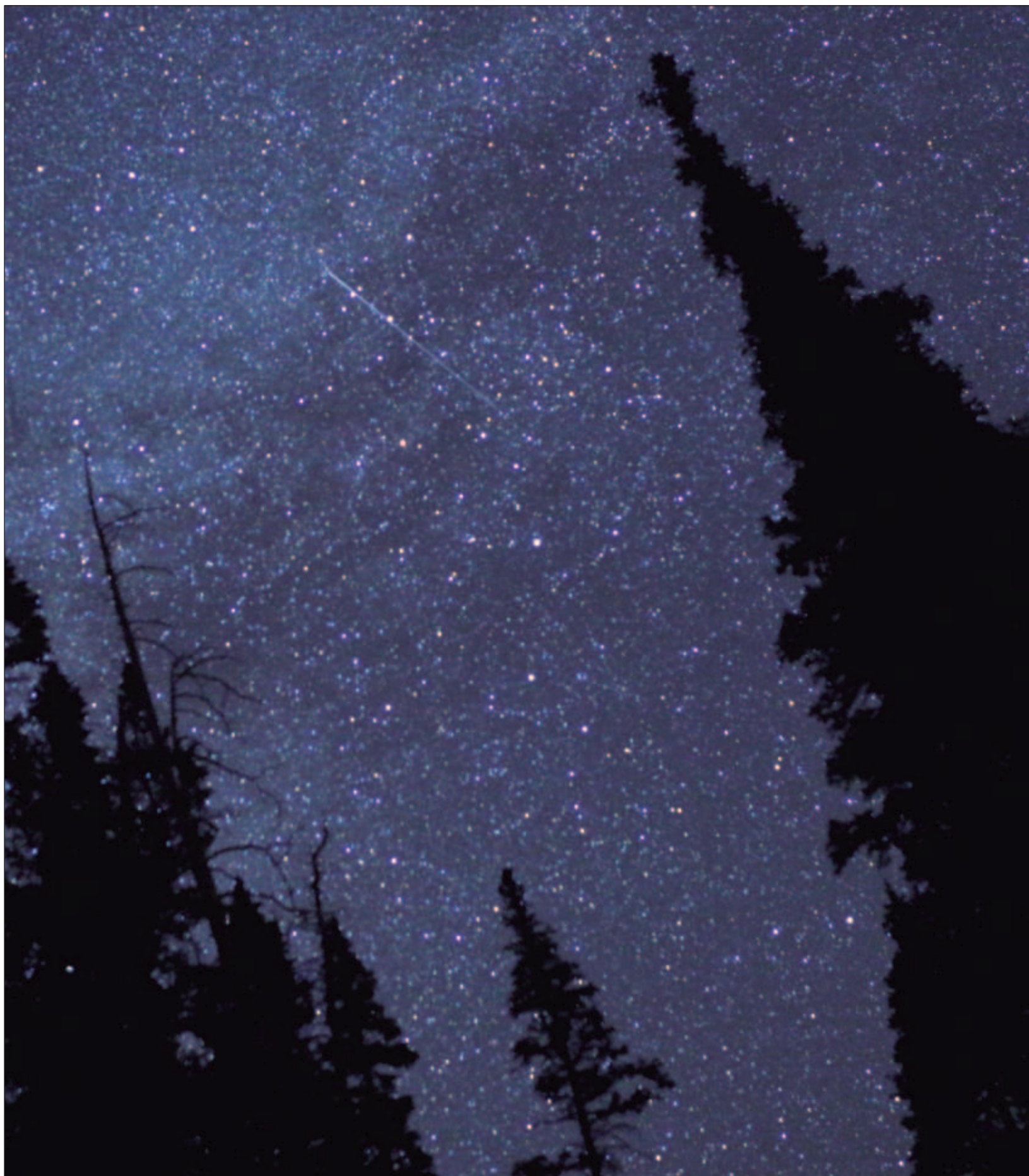
▲ Las deltas acuáridas del sur, fenómeno que se caracteriza por una actividad moderada, generando aproximadamente unos 25 meteoros por hora bajo condiciones óptimas de observación y que se extiende desde el 12 de julio hasta el 23 de agosto, tendrán su pico en el hemisferio norte entre el 30 y el 31 de julio, informa el Instituto Geográfico Nacional. Foto NASA
