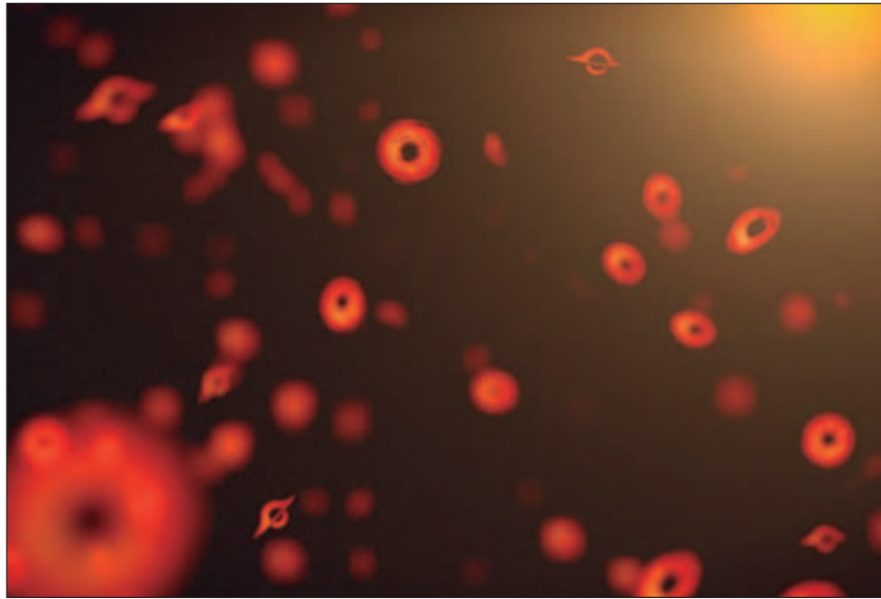
▲ A medida que el universo se expandió rápidamente después del Big Bang, es posible que algunas áreas del espacio fueran más densas que sus alrededores, lo que provocó que colapsaran y formaran agujeros negros primordiales o PBH. Foto NASA
